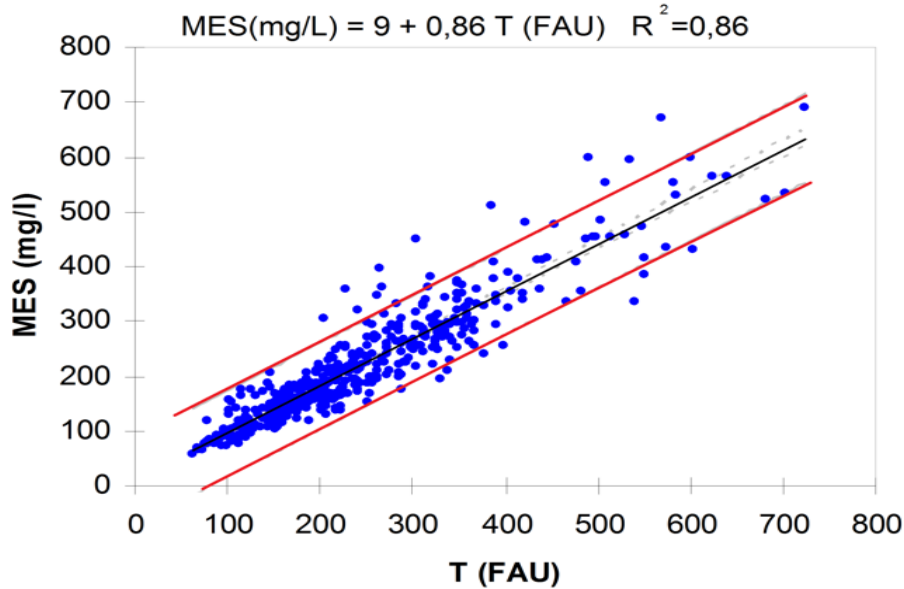
Figure 4 : relations turbidité- MES et incertitudes de prédiction associées (lignes rouges pleines). Les points bleus représentent les données utilisées pour construire ces relations et illustrent la qualité des ajustements.
