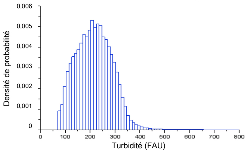
Figure 3: Distribution des turbidités instantanées
