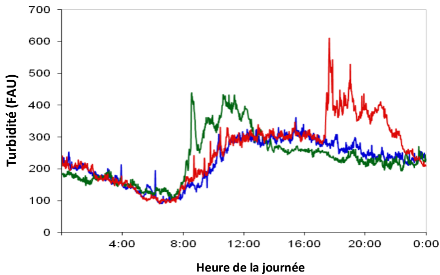
Figure 2: exemples d'enregistrement de turbidité (chaque couleur correspond à une journée, en bleu une journée de temps sec, en rouge et vert deux journées de temps de pluie)
